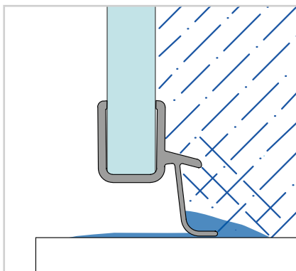
Bezrámové zástěny bez prahové lišty
