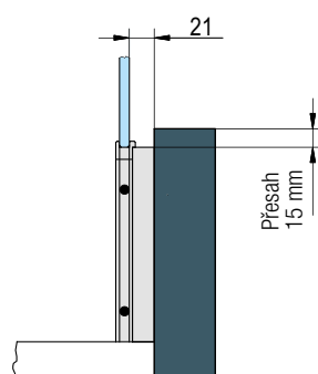
Detail A - pohled zředu
