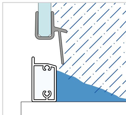
Rámové zástěny s rámovými profily
