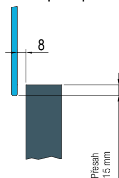
Detail A – pohled zepředu
