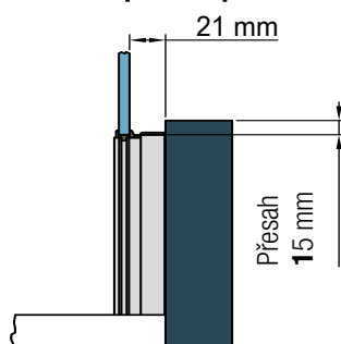
Detail A - pohled zepředu
