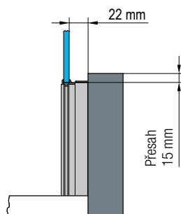
Detail A – pohled zepředu
