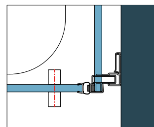
Detail A - půdorys
