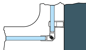
Detail A - půdorys
