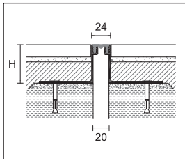
PBE/20 guma hladká
