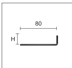
CPLB/2 základna perforovaná pro keramické dlažby
