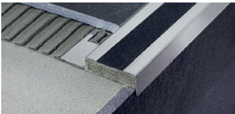
SIX/10 nerez ocel broušená AISI 304 - DIN 1.4301 + protiskluzový černý 25 mm
