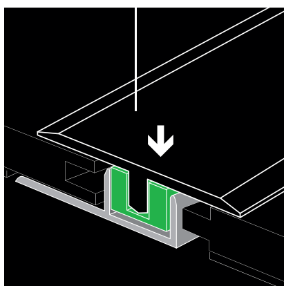
zatlačte vrchní profil na základnu
