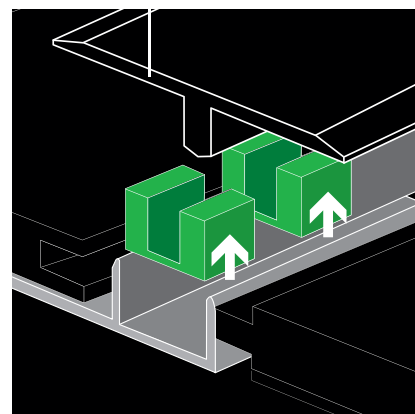
vložte klip pro vrchní profil
