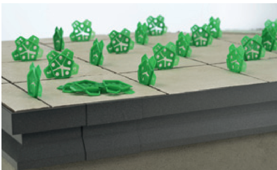
distanční rozpěrka
