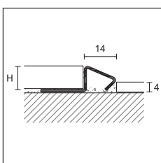
MIN/10 použití pro podlahy o rozdílné výšce
