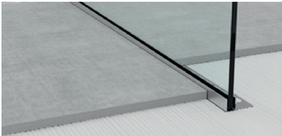
GPS1/DX/19 nerez ocel broušená AISI 304 DIN 1.4301
