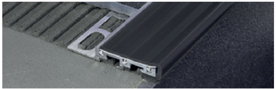
SB/10 hliník + PVC šedý tmavý
