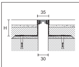
PBE/30 guma proužkovaná
