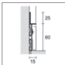
88/6 + 88/16L/A vložka z hliníku per LED
