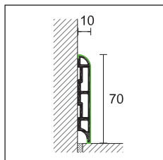
8605 potažené fólií Alcrom Plus
