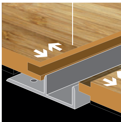
přiblížte podlahu k liště
