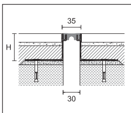
PBE/30 guma hladká
