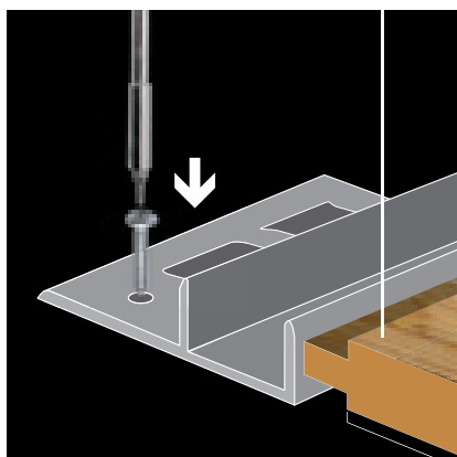
zafixujte základní hliníkový profil do podkladu šrouby nebo lepidlem
